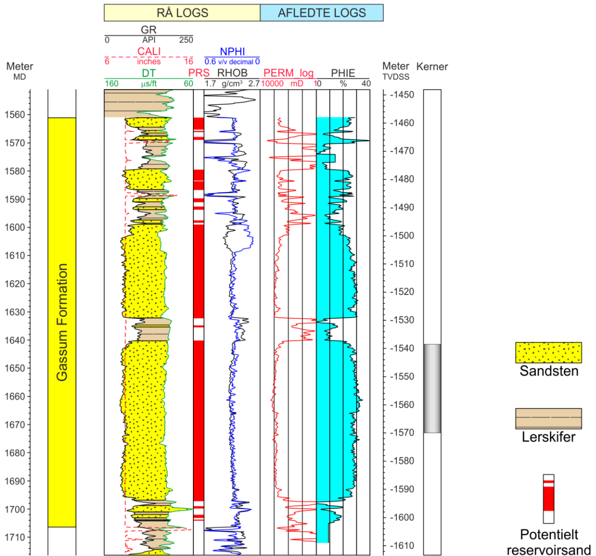
Figur 8: Petrofysisk log-tolkning af Gassum Formationen i Stenlille-19 inklusiv en tolkning af lithologien. Lithologi-kolonnen er afgrænset af gamma-ray (GR) og sonic (DT) loggene. Sektioner med Potentielt reservoirsand (PRS) er markeret med rødt fyld. Porøsitetsestimatet (PHIE) er fremhævet med lyseblåt fyld, og permeabilitets-estimatet (PERM_log) er plottet som en rød kurve. Logforkortelserne er forklaret i Tabel 5.4. Formationen er i boringen vist med dens vertikale tykkelse. MD: Målt dybde fra referencepunkt på boreplatform, TVDSS: Vertikale dybde under havniveau.
