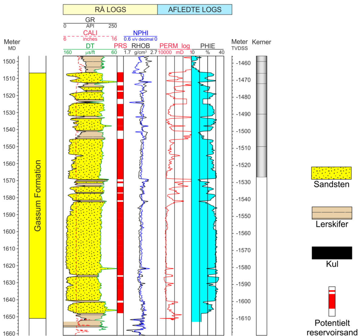
Figur 7: Petrofysisk log-tolkning af Gassum Formationen i Stenlille-1 inklusiv en tolkning af lithologien. Lithologi-kolonne er afgrænset af gamma-ray (GR) og sonic (DT) loggene. Sektioner med Potentielt reservoirsand (PRS) er markeret med rødt fyld. Porøsitetsestimater (PHIE) er fremhævet med lyseblå fyld, og permeabilitets-estimer (PERM_log) er plottet som en rød kurve. Logforkortelserne er forklaret i Tabel 5.4. Formationen er i boringen vist med dens vertikale tykkelse. MD: Målt dybde fra referencepunkt på boreplatform, TVDSS: Vertikale dybde under havniveau.
