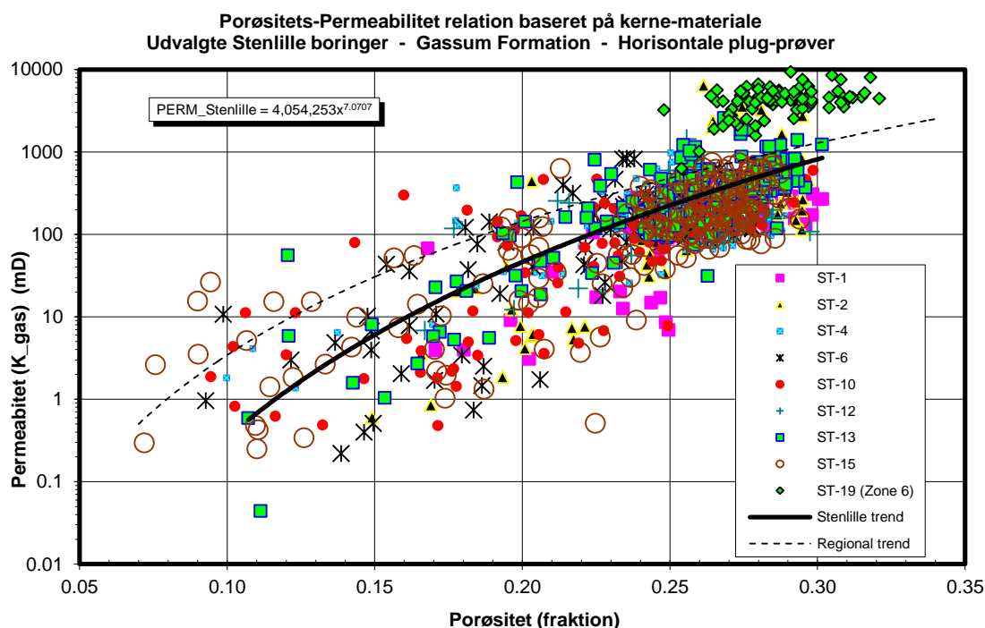
Figur 9: Generaliseret sammenhæng mellem porøsitet og permeabilitet estimeret ud fra kerne-analyse data, dvs. målinger af porøsitet og permeabilitet på små plug prøver. Den fuldt optrukne linje repræsenterer tendenslinjen for Stenlille-1 til -15 datapunkterne, der stammer fra den øvre del af Gassum formationen (Zone 1–5). Data fra Stenlille-19 stammer fra den nedre del af Gassum Formationen (Zone 6). Den stiplede linje repræsenterer GEUS' regionale model og antages, ud fra en gennemsnitsbetragtning, at være gældende for Slagelse-området.
