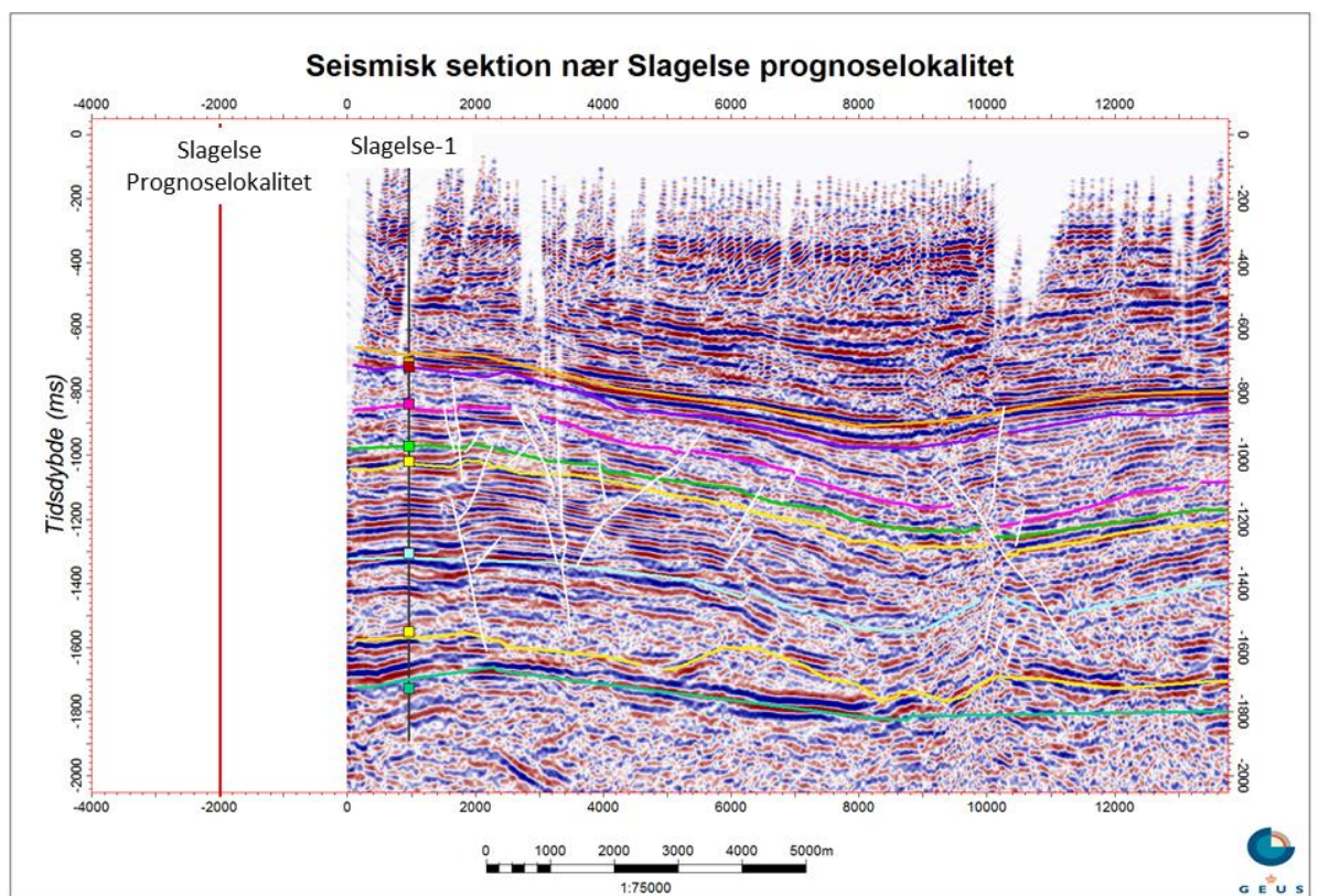
Figur 5: Seismisk profil baseret på den seismiske linje 72/001, der passerer syd om prognoselokaliteten i en afstand af ca. 5 km (Figur 3 og 4). Prognoselokalitet er projiceret vinkelret ind for enden af profilet og er markeret med en rød, lodret streg. Profilet viser, at der forekommer flere mindre forkastninger (markeret med hvide streger) gennem Gassum Formationen i området. Det fremgår også af profilet, at der i Slagelse-området forekommer mindre saltstrukturer i Zechstein Gruppen. Dybde er angivet som seismisk to-vejs-tid i millisekunder. Oppefra og ned er følgende tolkede horisonter vist på figuren (også markeret ved farvede rektangler i Slagelse-1 boringen): Basis af Kalkgruppen (orange), Top Fjerritslev Fm (lilla), Top Gassum Fm (lyserød), Top Vinding Fm (lysegrøn), Top Oddesund Fm (gul), Top Bunter Sandsten Fm (lyseblå), Top Zechstein Fm (gul) og Top Pre-Zechstein Fm (turkisgrøn). På figuren fremgår endvidere de nominelle tidsdybder af de tilsvarende lithologiske grænser i Slagelse-1 brønden.
