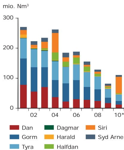
fig. 5.4 Flaring
