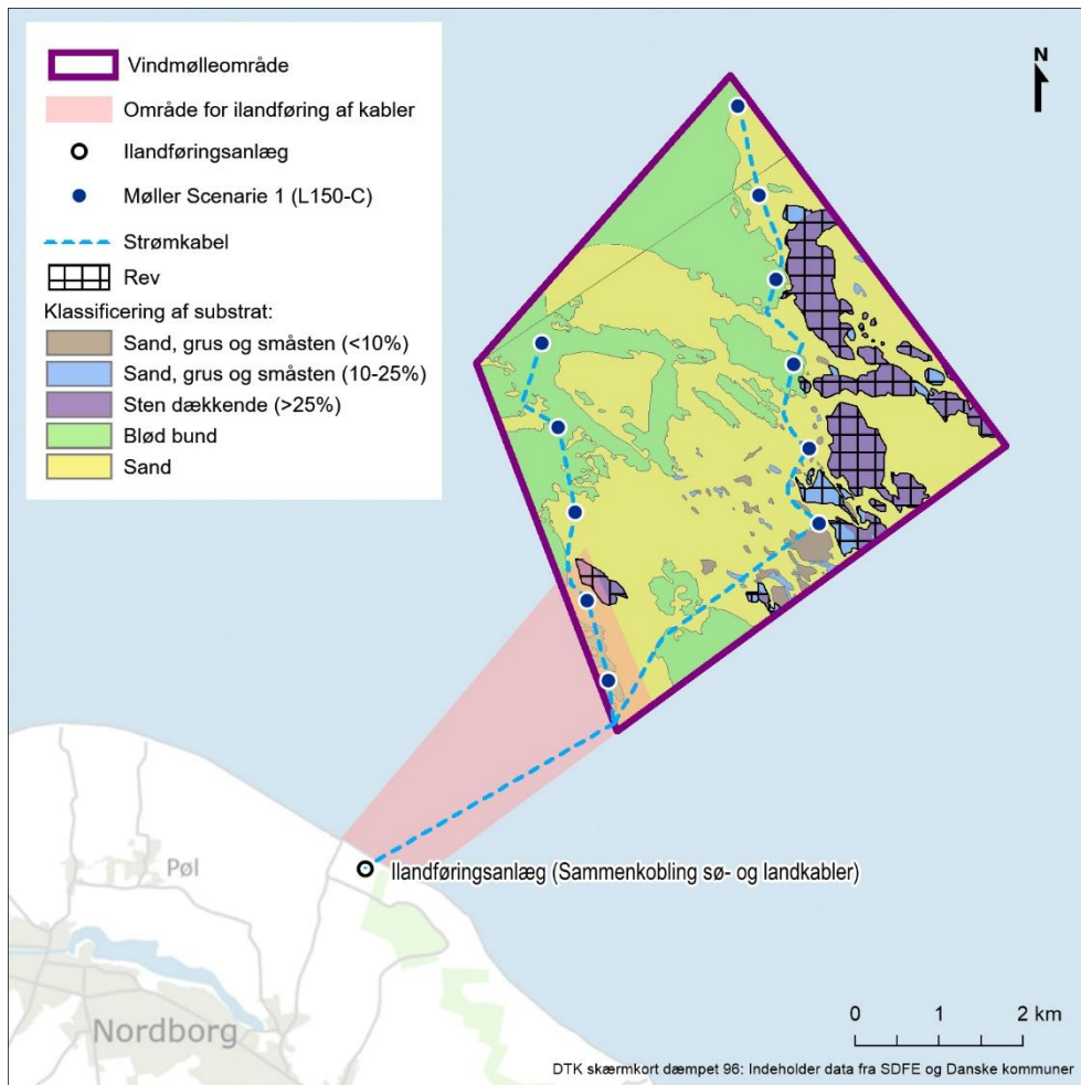
Figur 1 Layout over projektområdet og korridoren for ilandføringskablerne
