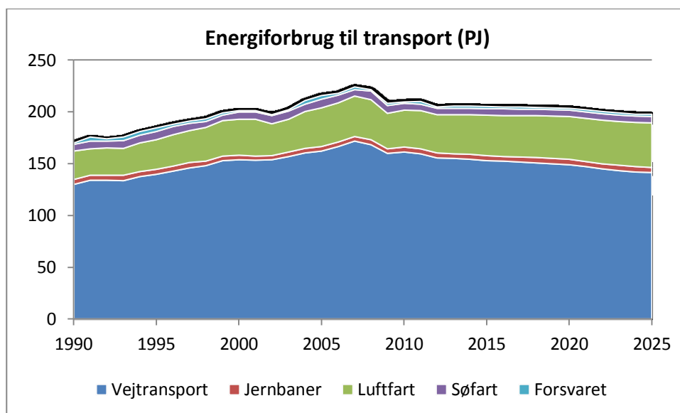
Figur 21: Transportsektorens energiforbrug fordelt på transportmidler (PJ)
