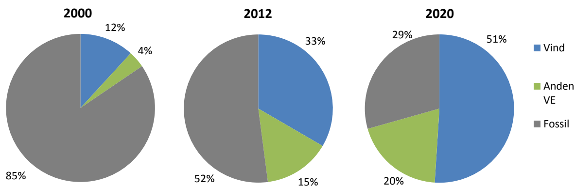
Figur 3: Danmarks elforbrug (inkl. nettab) fordelt på typer af kilder, elhandelskorrigeret, fossil dækker over kul, olie, naturgas samt ikke bio-nedbrydeligt affald. Elproduktionen for 2020 er vist for middelskønnet for kvoteprisen.
