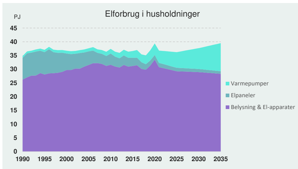
Figur 1: Elforbrug i husholdningerne fordelt på slutanvendelser .
