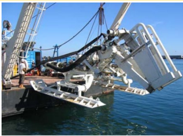
Pharos Q1000
