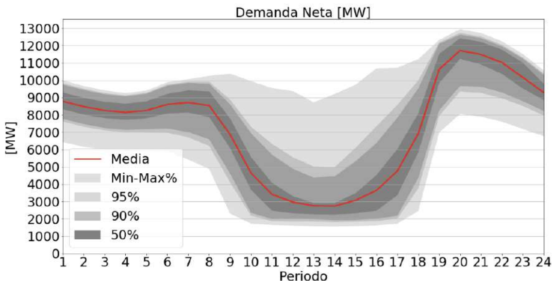
Figura 7. Proyección de la demanda neta horaria de energía de la “curva del pato” para Colombia en 2030 [40].
