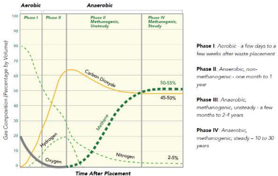
Figura 93. Generación de Gas de Relleno Sanitario (LFG) y cambios a lo largo del tiempo [4].
