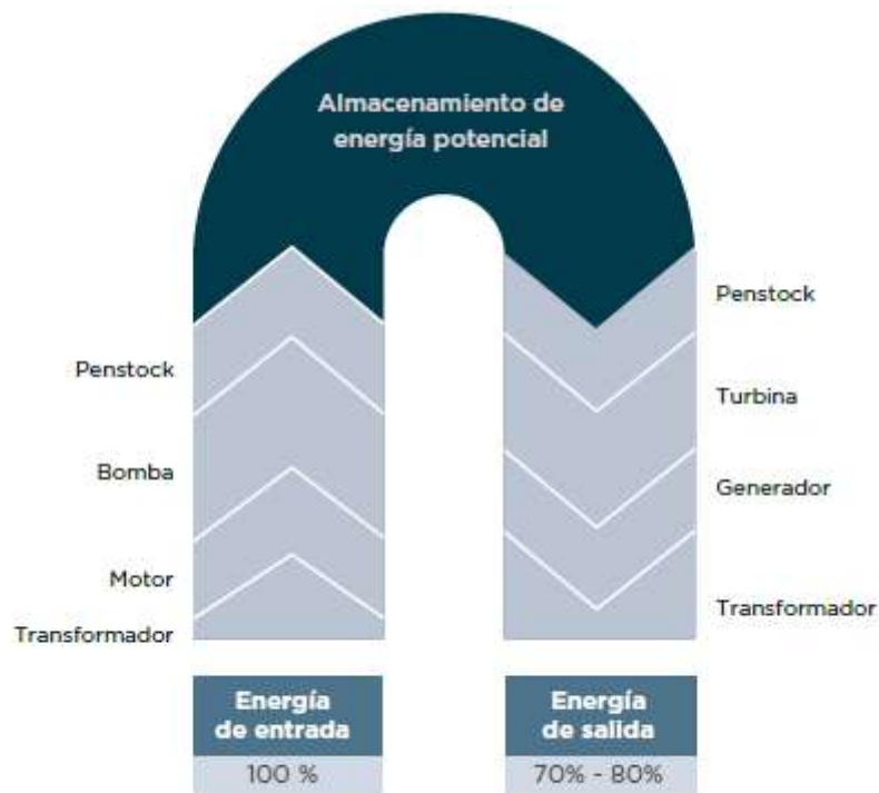
Figura 129. Eficiencia del ciclo hidroeléctrico de bombeo [1].
