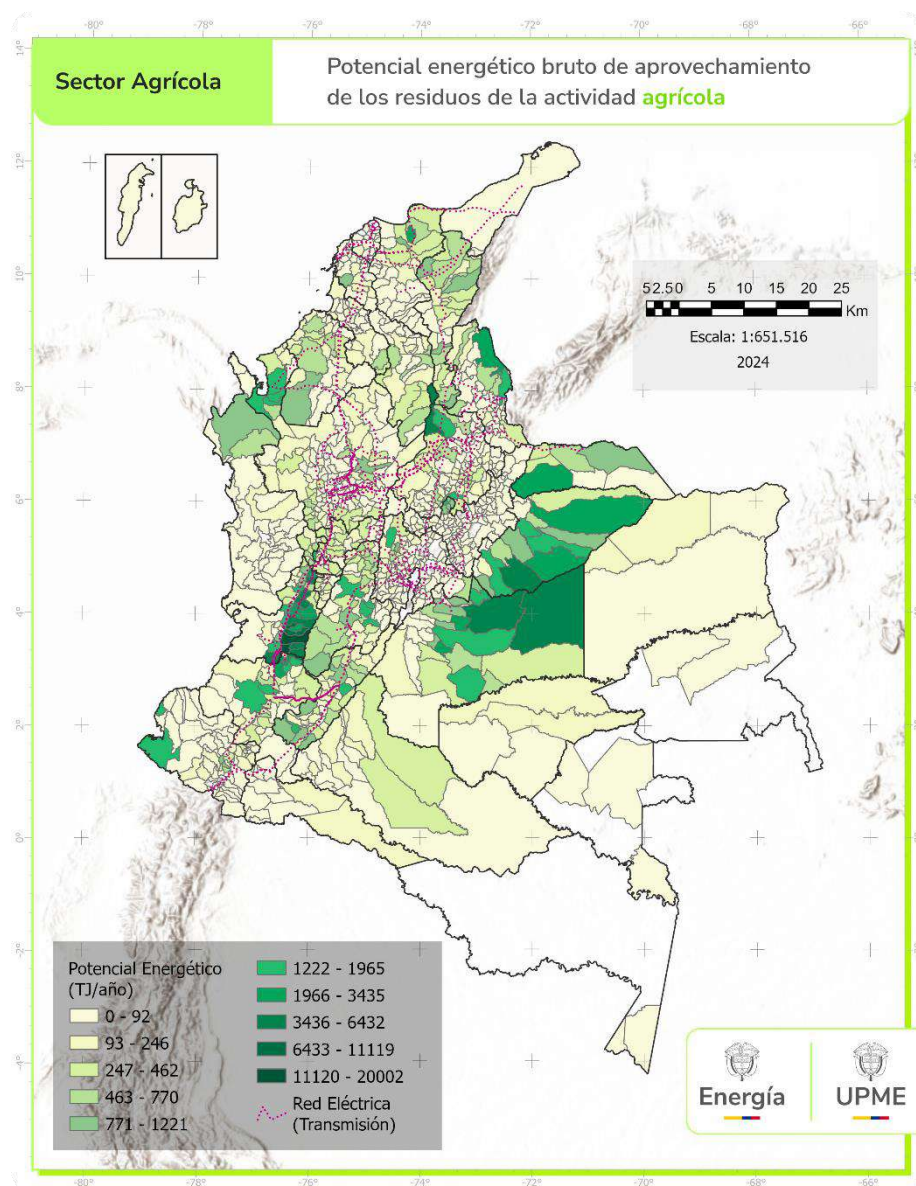
Figura 65. Potencial Energético de la Biomasa Residual Agrícola [9].
