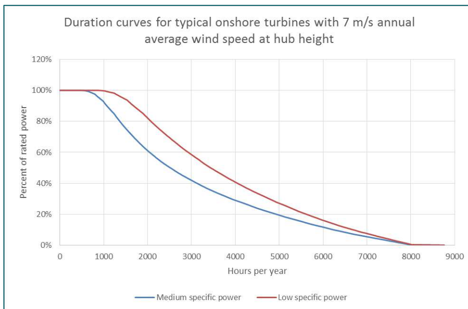
Figura 20. Curvas de duración basadas en las turbinas V117 de 3,3 MW ( 307 \text{ W/m}^2 ) y V126 de 3,3 MW ( 265 \text{ W/m}^2 ) de energía eólica terrestre situadas en Dinamarca [2]. Faltan datos empíricos para Colombia debido a que no hay cifras operativas representativas a partir de 2024.
