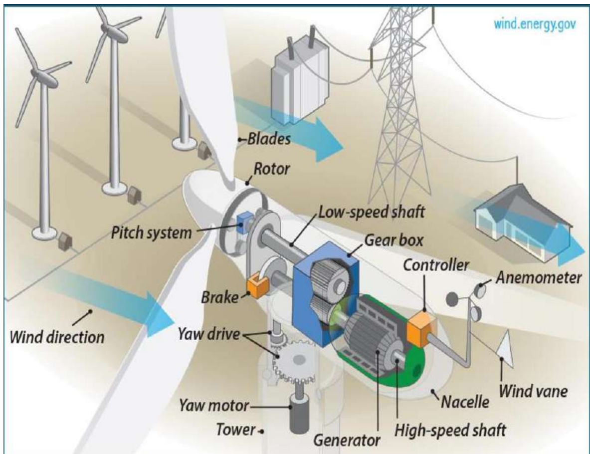
Figura 18. Tecnología general de turbinas y sistema eléctrico [1].
