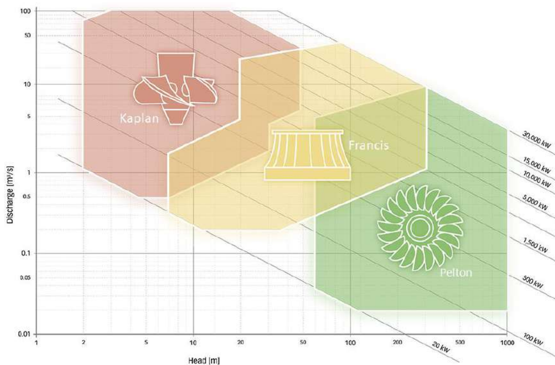
Figura 42. Cuadro de aplicaciones de las turbinas hidroeléctricas [5].
