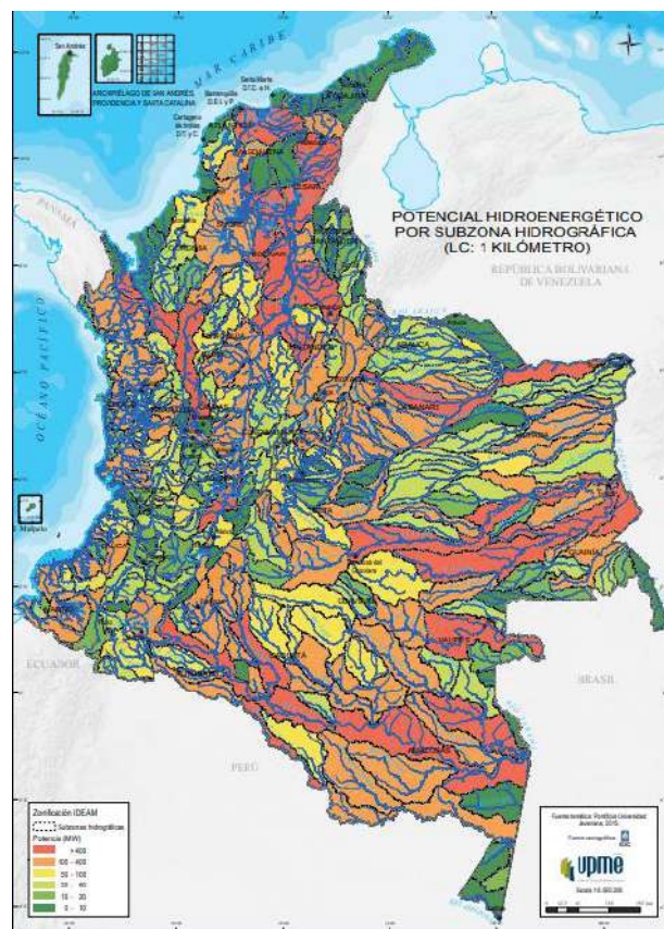
Figura 44. Potencial hidroeléctrico por zona subhidrográfica en Colombia [7].
