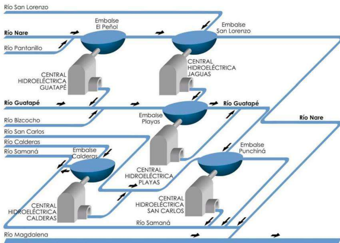
Figura 40. Sistema de la cadena hidroeléctrica Nare-Guatapé [2].
