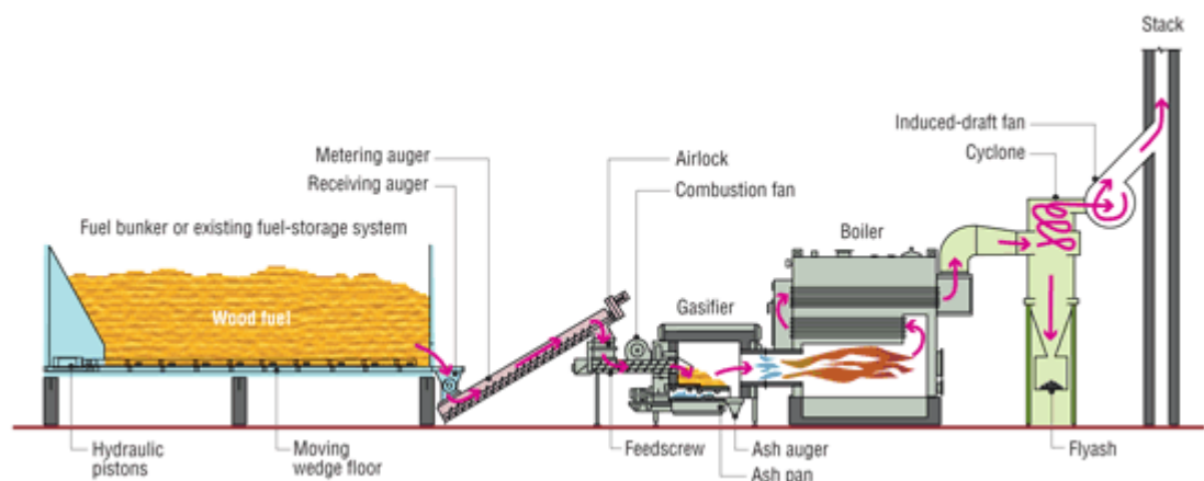
Figura 62. Caldera de biomasa de lecho fijo [4].
