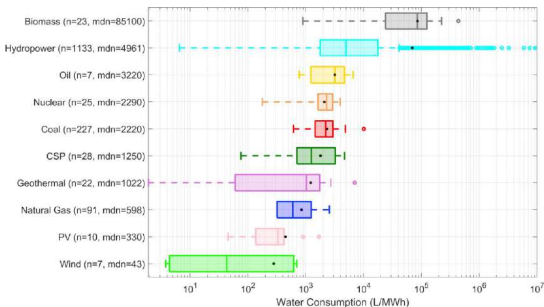
Figura 111. Comparación del consumo de agua de las fuentes de energía [24].
