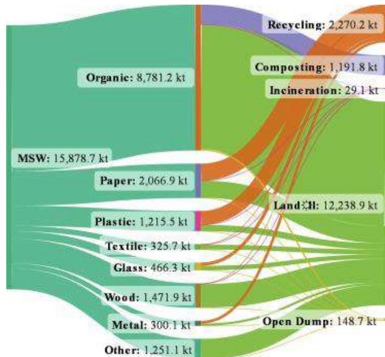
Figura 95. Diagrama de Sankey de creación y eliminación de residuos sólidos urbanos en Colombia [9].
