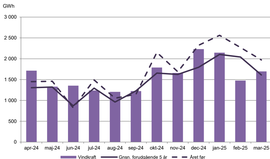
Figur 11. Vindkraftproduktion [GWh]
