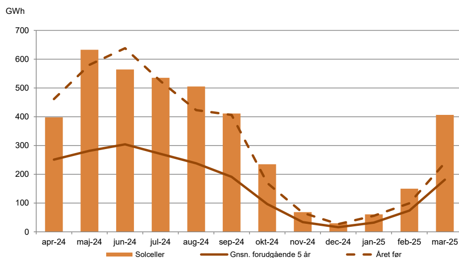
Figur 12. Solkraftproduktion [GWh]
