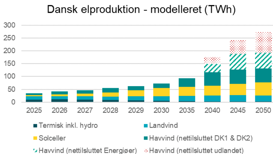
Figur 2: Samlet elproduktion nettilsluttet Danmark (inkl. energiøer), samt elproduktion fra havvind på dansk territorie nettilsluttet udlandet
