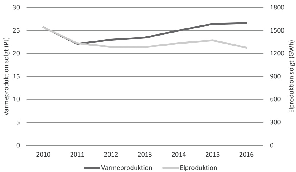
Figur 15: Den samlede el- og varmeproduktion fra 2010 – 2016, dedikerede forbrændingsanlæg.
