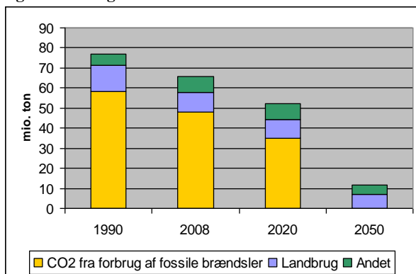
Figur: drivhusgasemissioner 1990-2050.
