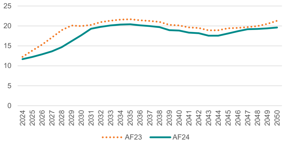
Figur 9: Samlet produktion fra landvind i AF23 og AF24 (TWh, primo året)
