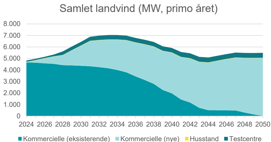
Figur 6: Samlet landvindkapacitet i AF24 (MW, primo året)
