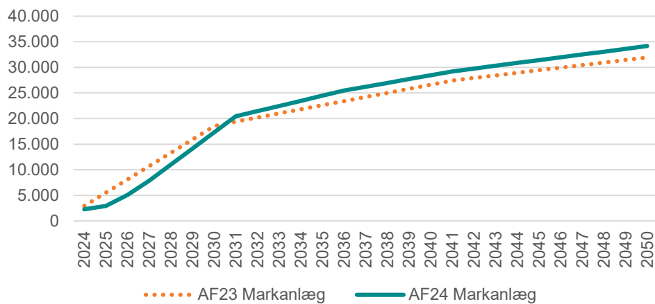
Figur 3: Solcellekapacitet for markanlæg i AF23 og AF24 (MW, primo året)
