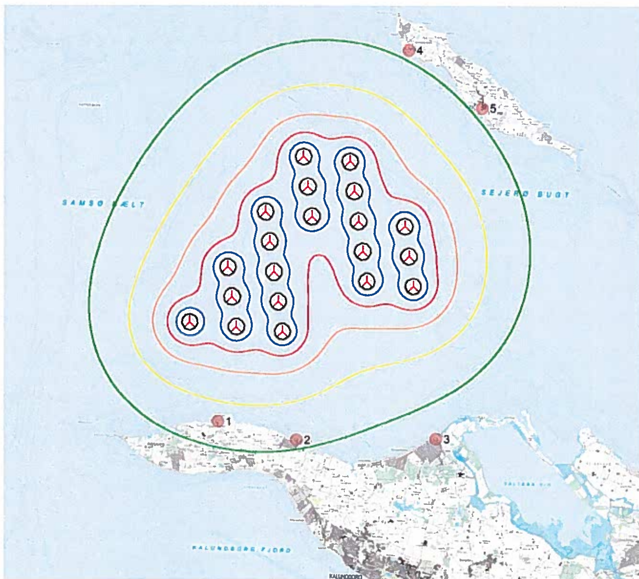
Figur 20-41. 10 MW havmøller ved 6 m/s. Grænseværdien er 42 dB(A) ved enkeltliggende boliger og 37 dB(A) ved områder til støjfølsom arealanvendelse, herunder boligområder og sommerhusområder. Gul=32dB. Grøn=27dB
